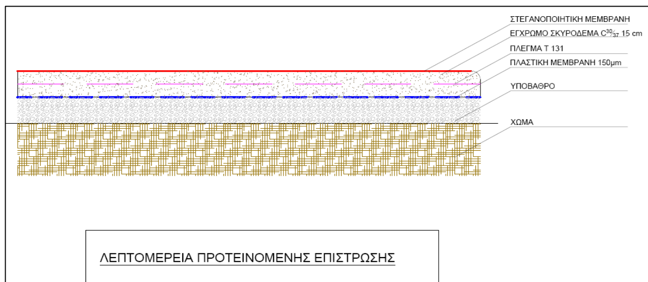
Εικ.3 Σχέδιο κατασκευαστικής λεπτομέρειας.
